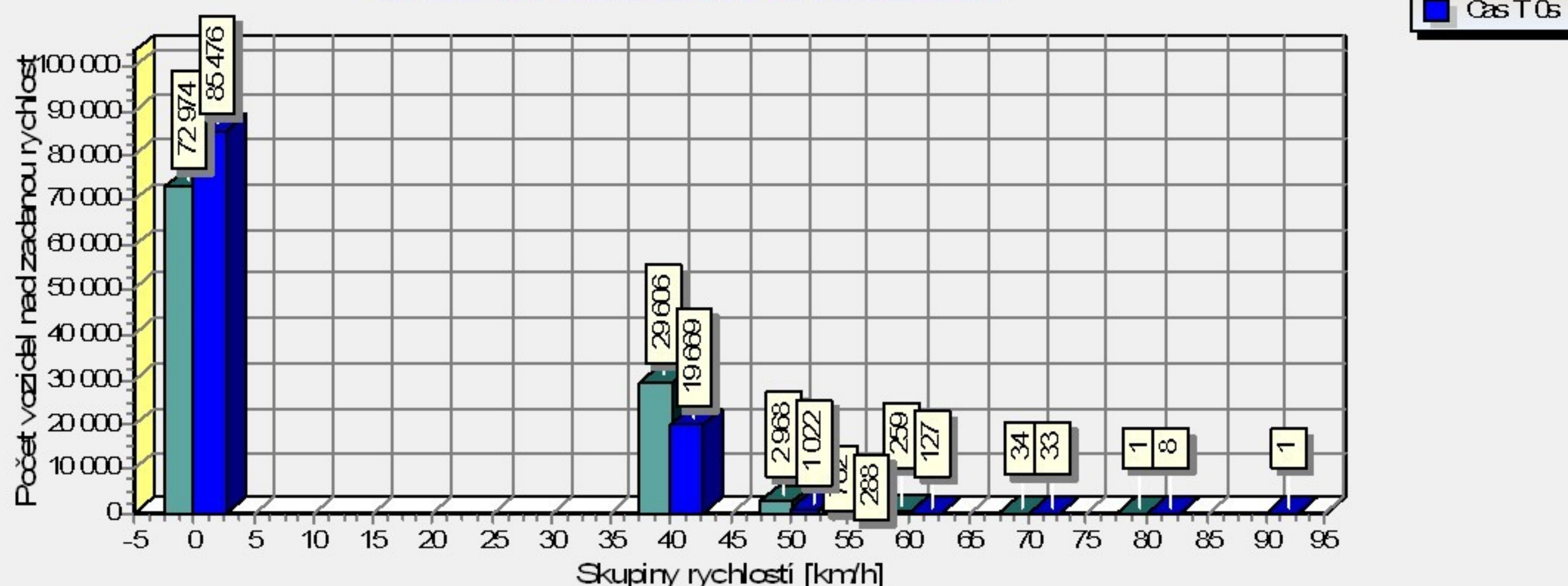
Graf rychlosti vozidel před zařízením v časech T 0s a T-5s za období od 01.12.22 00:00 do 31.12.22 23:59
