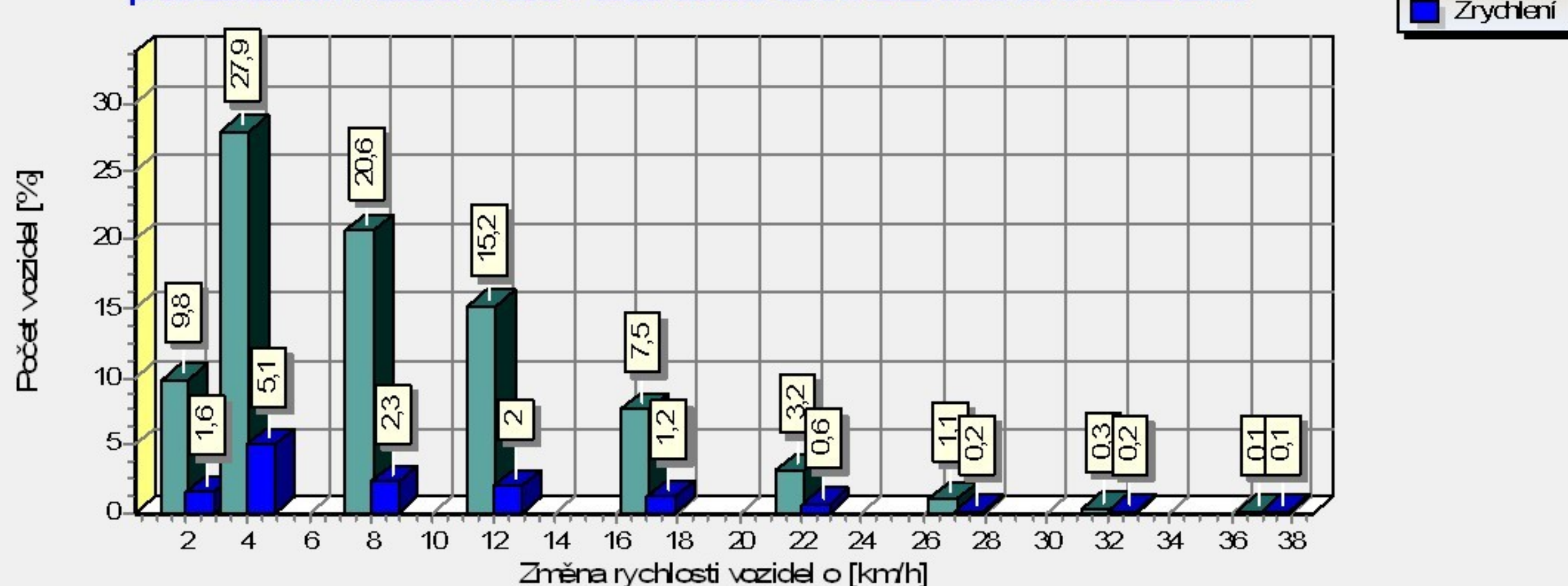
Graf velikosti změny rychlosti vozidel před zařízením v časech T 0s a T-5s za období od 01.12.22 00:00 do 31.12.22 23:59
