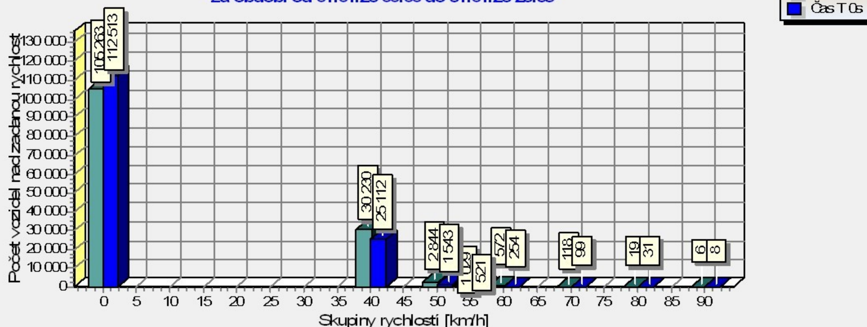
Graf rychlosti vozidel před zařízením v časech T 0s a T-5s za období od 01.01.23 00:00 do 31.01.23 23:59
