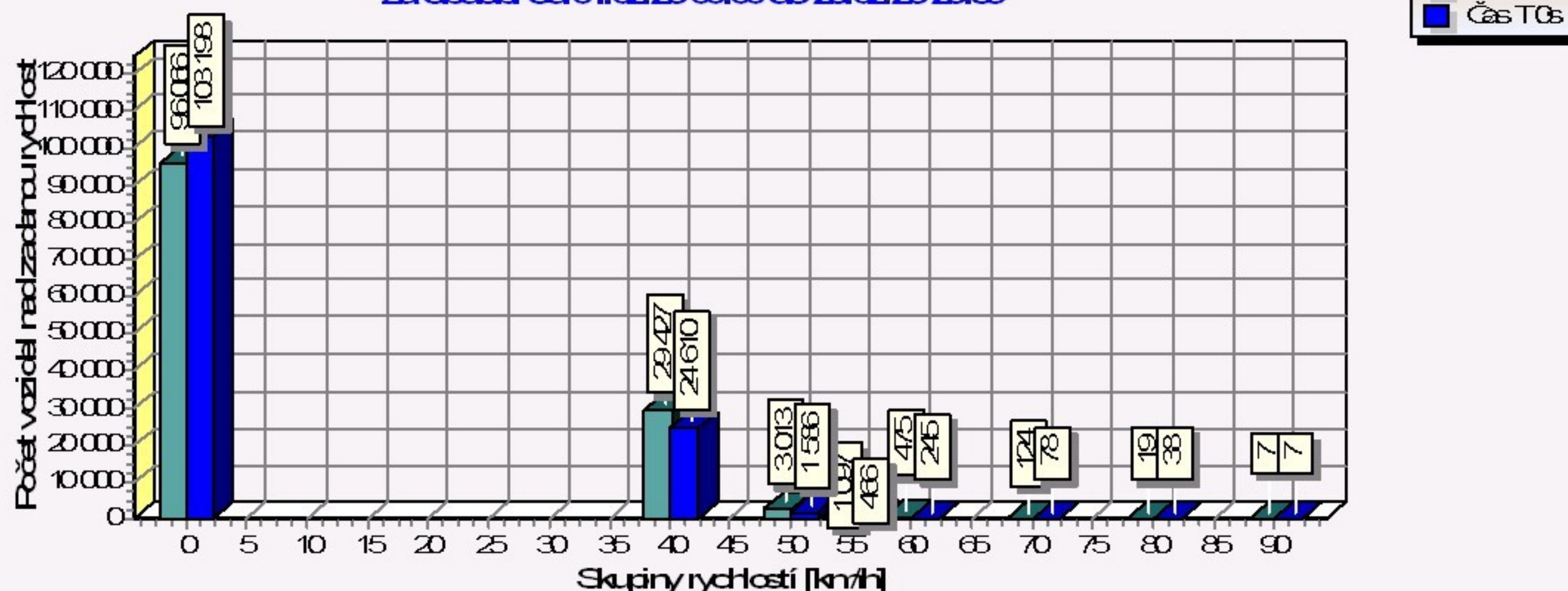
Graf rychlosti vozidel před zařízením v časech T0 a T5s za období od 01.02.23 00:00 do 28.02.23 23:59
