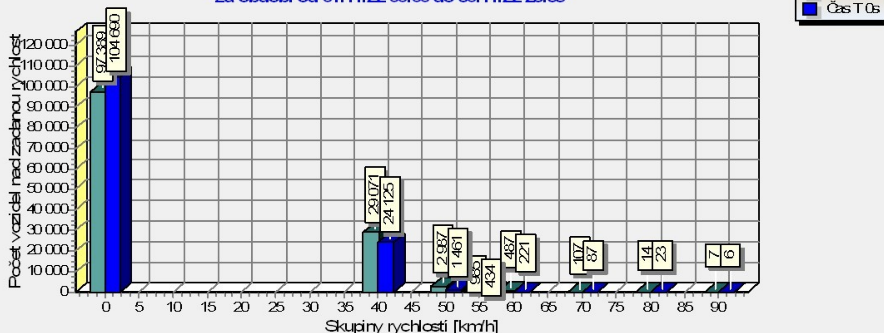
Graf rychlosti vozidel před zařízením v časech T 0s a T-5s za období od 01.11.22 00:00 do 30.11.22 23:59
