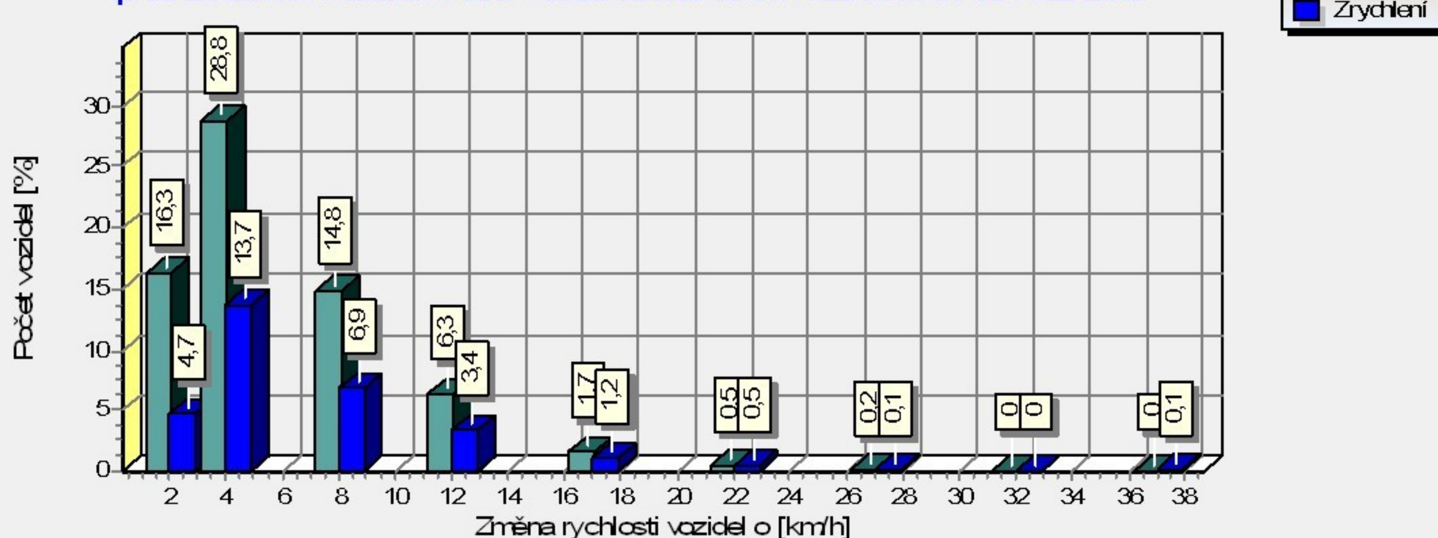
Graf velikosti změny rychlosti vozidel před zařízením v časech T 0s a T-5s za období od 01.11.22 00:00 do 30.11.22 23:59
